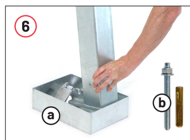
a) Bodenplatte für Fundamente / Ground plate for foundations b) Verbundanker (8 Stück) / Ground anchor (8 pcs)
