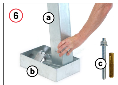
a) Abnehmbare Bodenhülse / Removable socket b) Bodenplatte für Fundamente / Ground plate for foundations c) Verbundanker (8 Stück) / Ground anchor (8 pcs)
