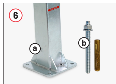
a) Bodenhülse für Fundamente / Bolt-down socket b) Verbundanker (8 Stück) / Ground anchor (8 pcs)
